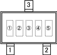
SOT-23(TO-236)
