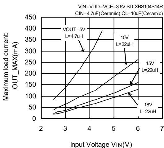
(4) 最大出力電流－入力電圧特性例
