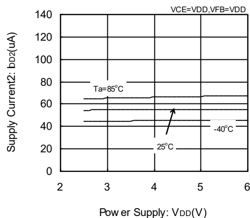
(7) 消費電流 2－入力電圧特性例
