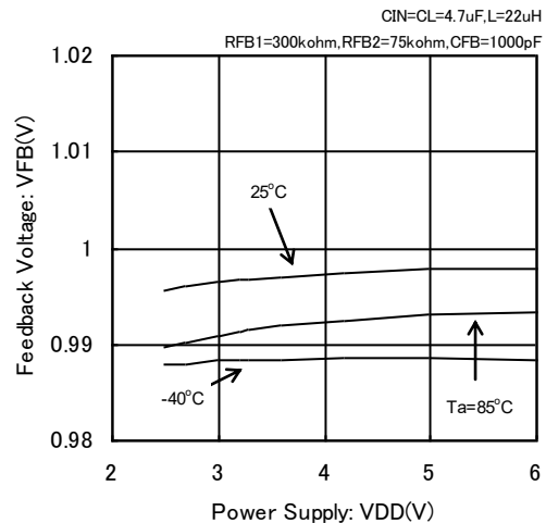
(13) FB 制御電圧—入力電圧特性例
