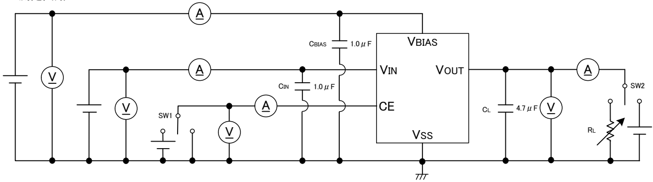
測定回路 1
