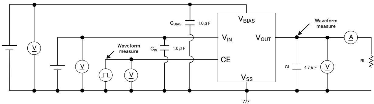
測定回路 3
