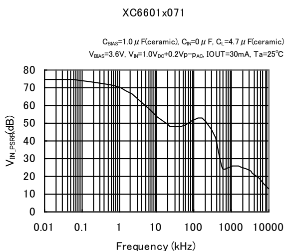
(16) 入力電圧リップル除去率特性例
