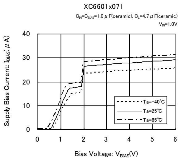
(5) バイアス電流-バイアス電圧特性例
