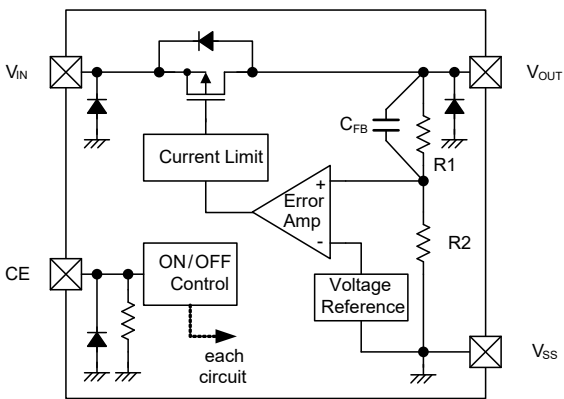
3) XC6501 シリーズ C タイプ
