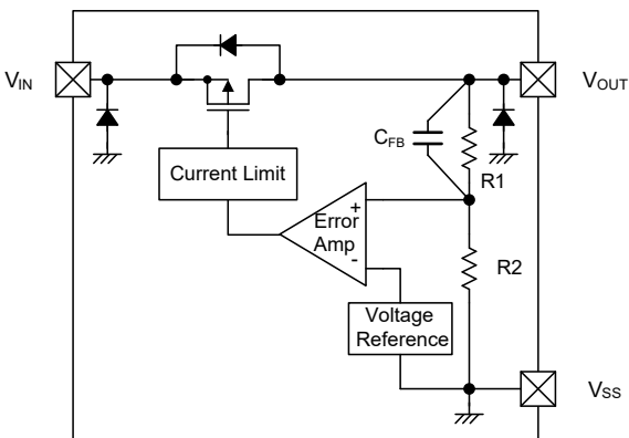
5) XC6501 シリーズ P タイプ
