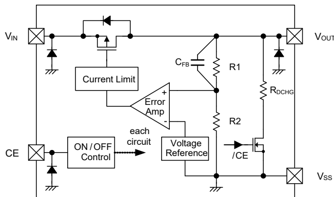
XC6501 シリーズ B タイプ
