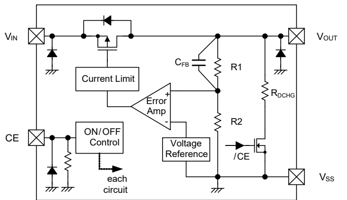
4) XC6501 シリーズ D タイプ
