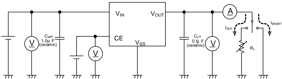
測定回路 ①
