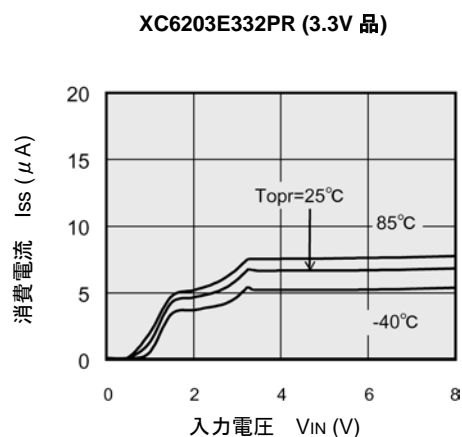
(4) 消費電流－入力電圧
