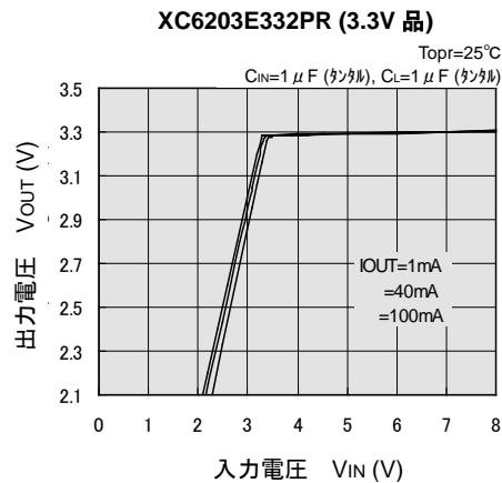
(2) 出力電圧－入力電圧
