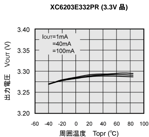
(5) 出力電圧－周囲温度
