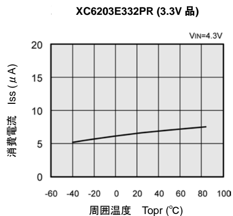
(6) 消費電流－周囲温度
