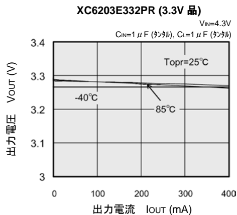
(1) 出力電圧－出力電流
