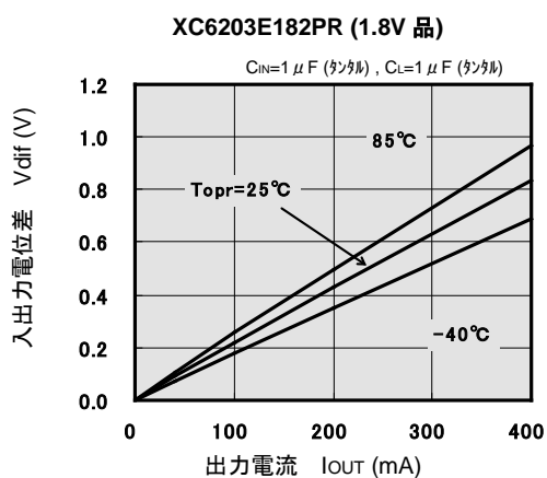
(3) 入出力電位差—出力電流
