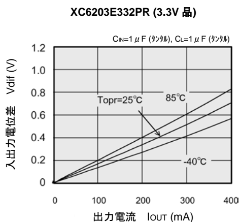
(3) 入出力電位差－出力電流
