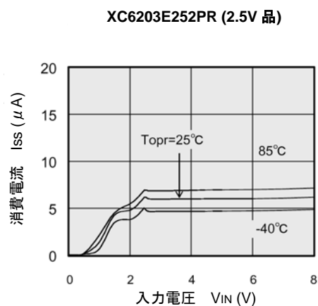
(4) 消費電流—入力電圧
