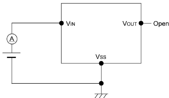
測定回路図①：消費電流
