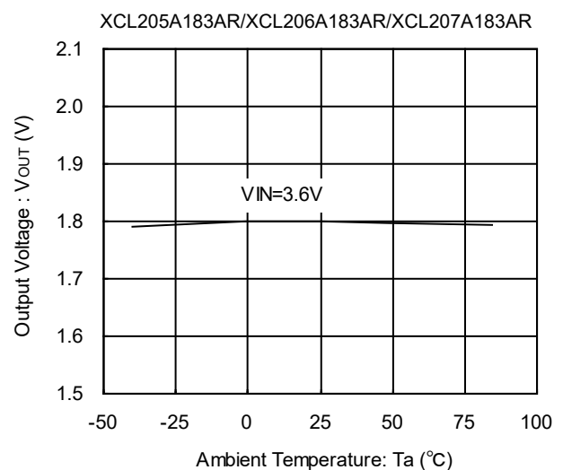
(6) 出力電圧 - 周囲温度
