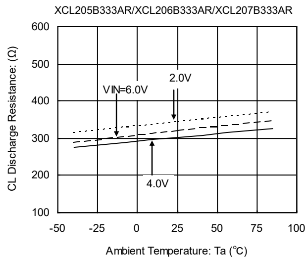
(14) CL 放電抵抗 - 周囲温度
