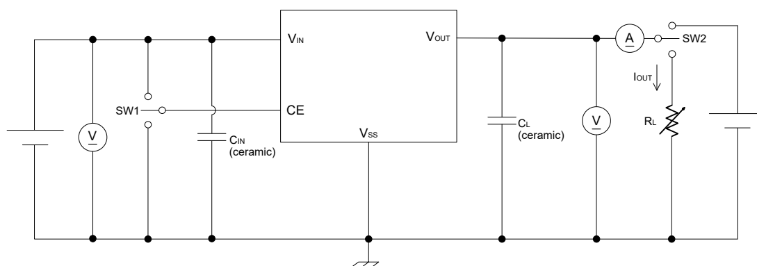
2)測定回路図②
