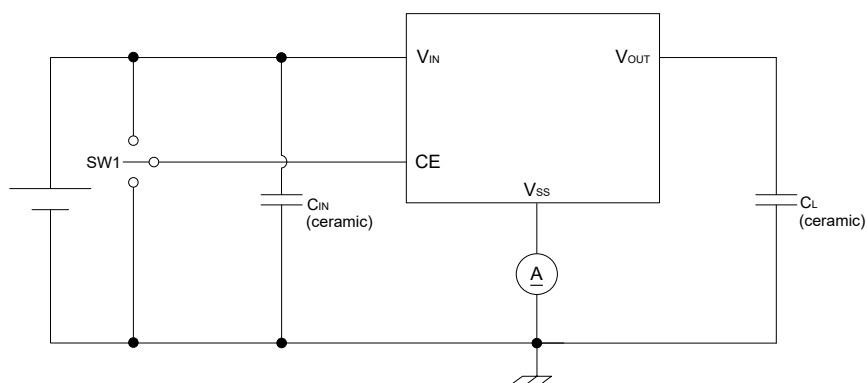
3)測定回路図③
