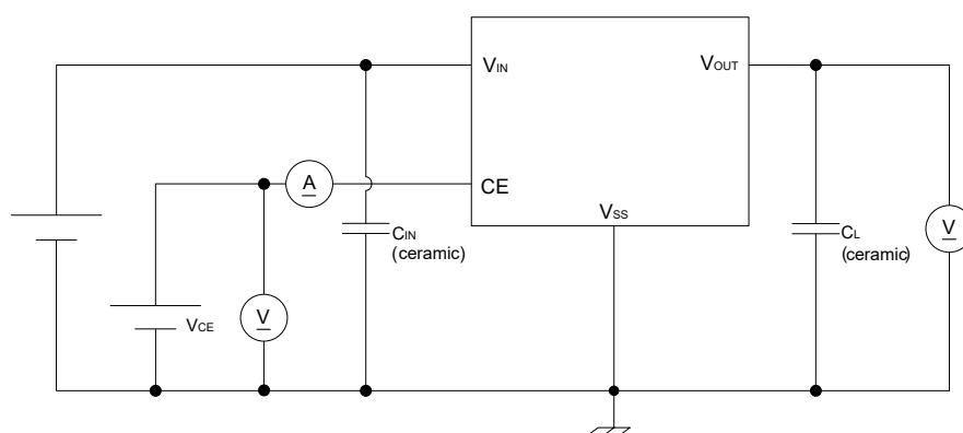
4)測定回路図④
