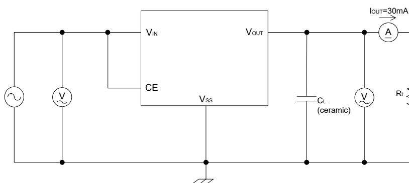
3)測定回路図③
