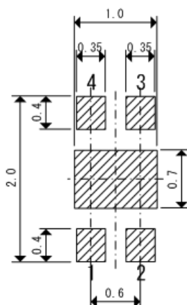
● USP-4 参考パターンレイアウト
