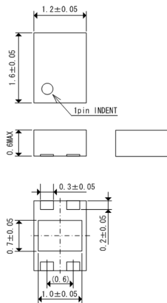
● USP-4 外形図 (unit:mm)
