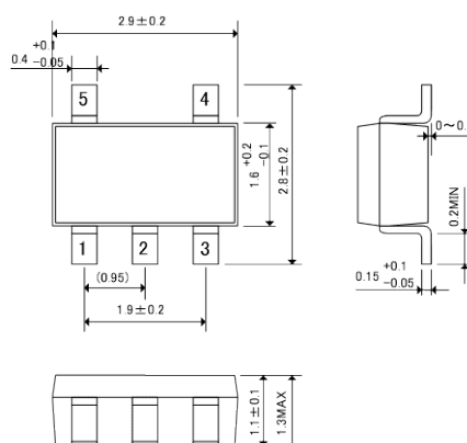
● SOT-25 外形図 (unit:mm)
