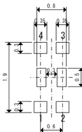
● USP-4 参考メタルマスクデザイン
