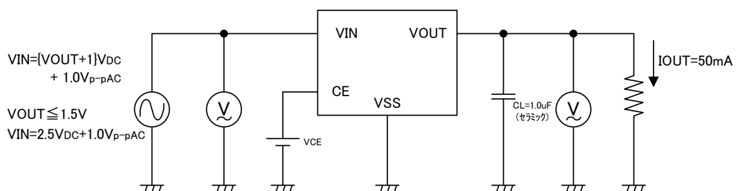
測定回路 ④
